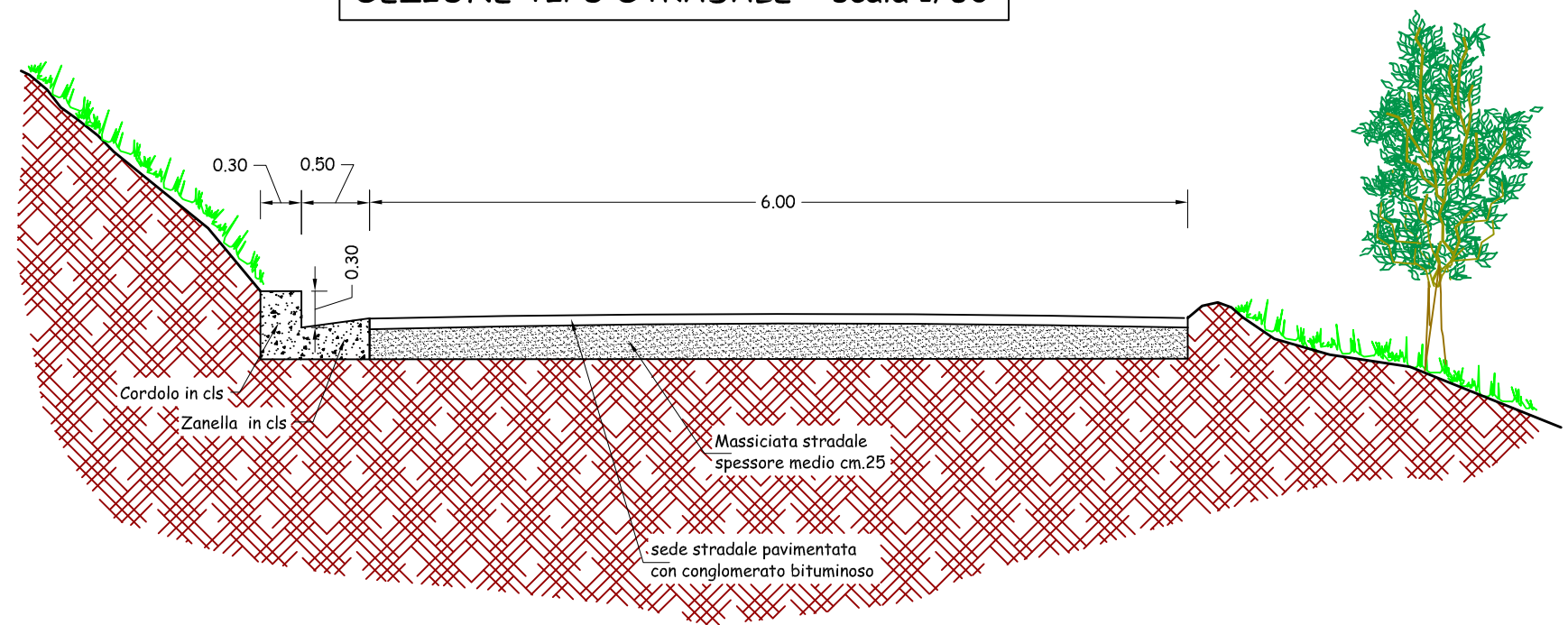
SEZIONE TIPO STRADALE scala 1/50
